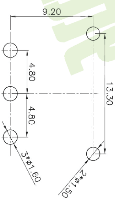
P.C.B layout
